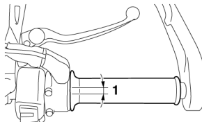
1. Folga da manopla do acelerador
