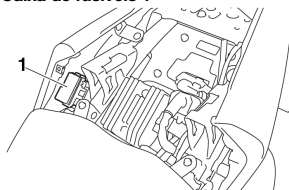
Caixa de fusíveis 1
