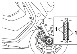
1. Indicador de desgaste da pastilha de freio
