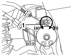
1. Parafuso de ajuste da marcha lenta
