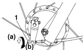
1. Porca de ajuste
